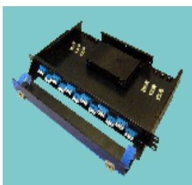
前面トレーユニット実装イメージ
